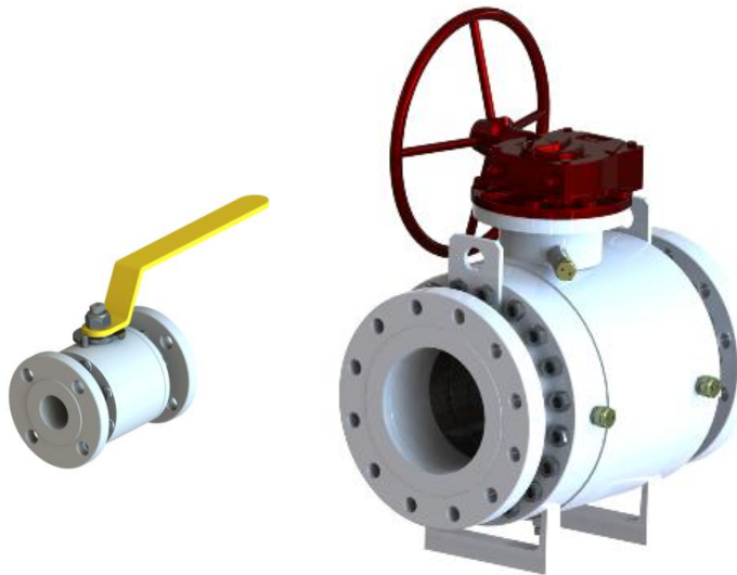
VALVOLA A SFERA SPLIT BODY (DUE O TRE PEZZI) PN 10-420, CLASSE 150-2500
