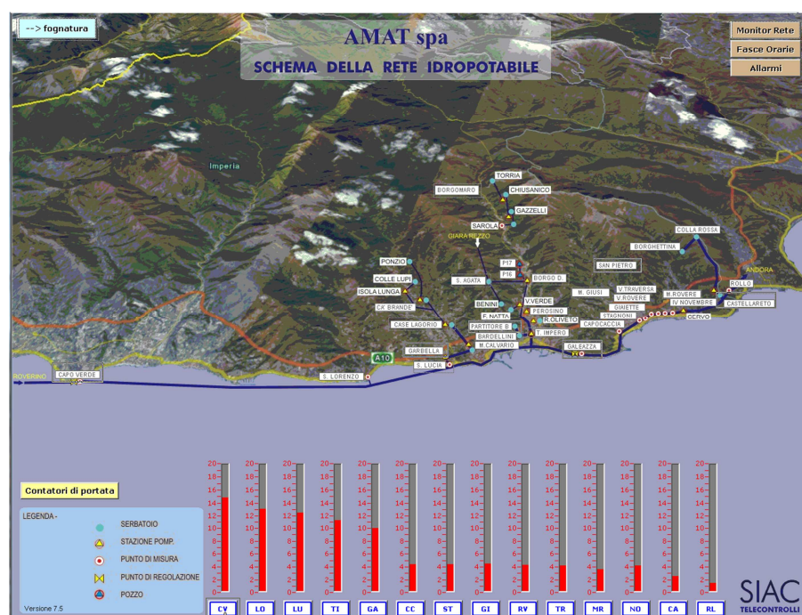
1.Schema della rete idropotabile
