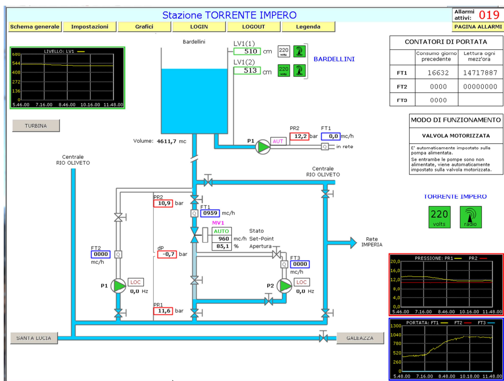
4. Dettaglio dell'impianto Stazione Torrente Impero
