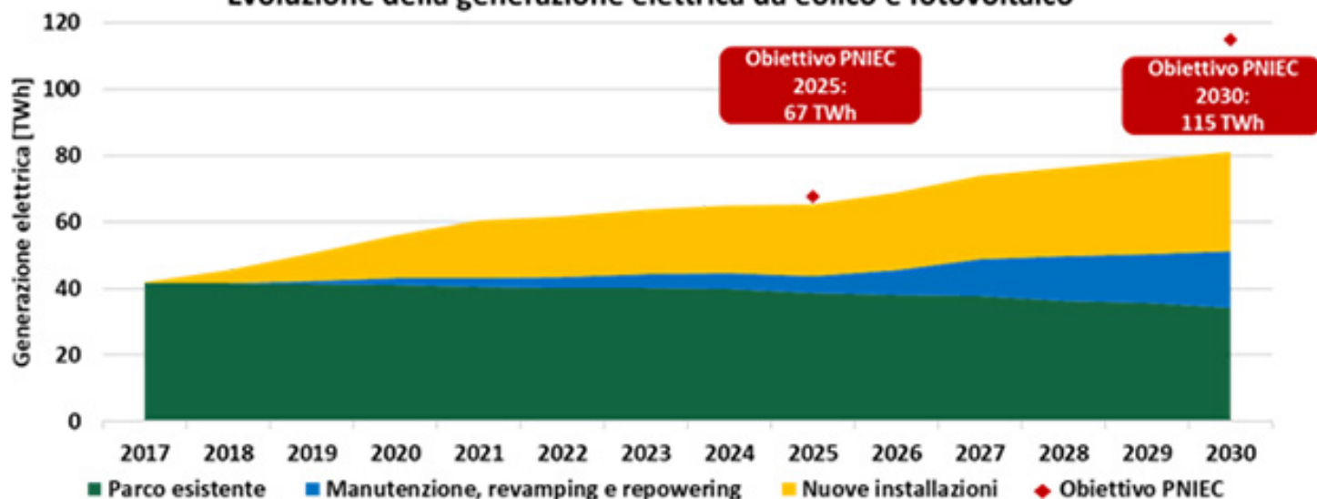
Evoluzione della generazione elettrica da eolico e fotovoltaico
