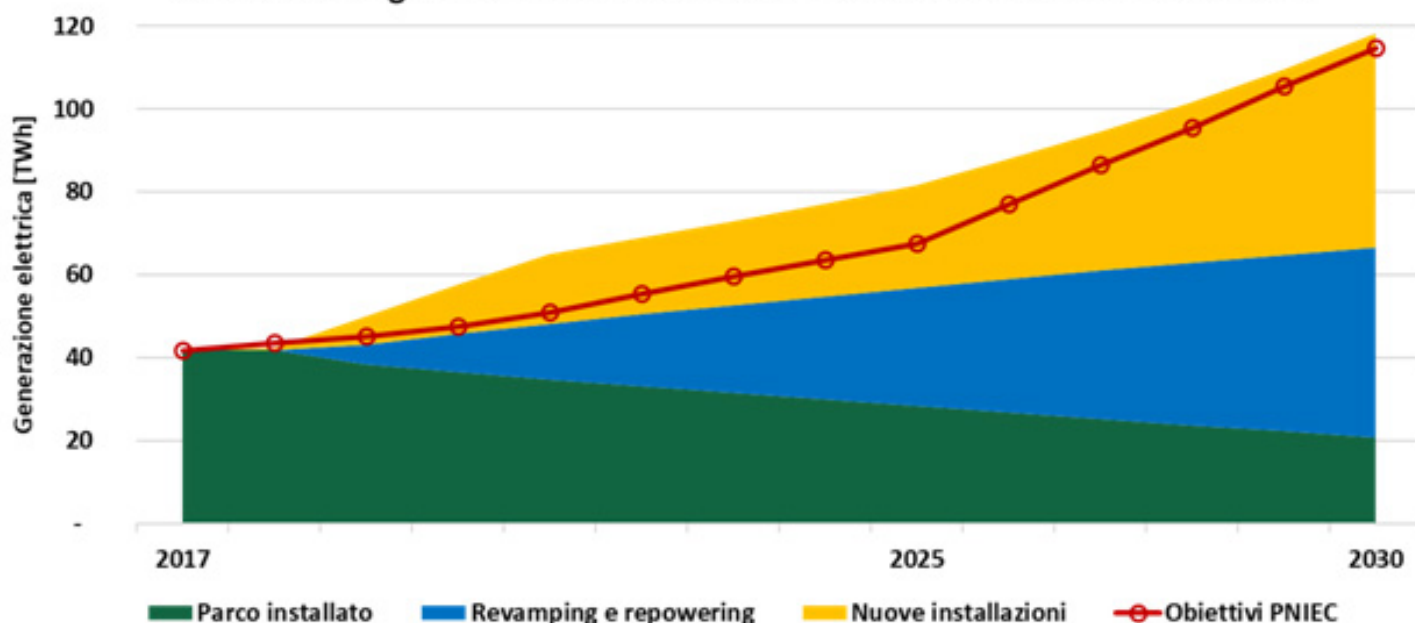
Evoluzione congiunta di eolico e fotovoltaico nello scenario «desiderabile 2»
